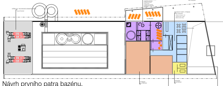
Návrh prvního patra bazénu.
