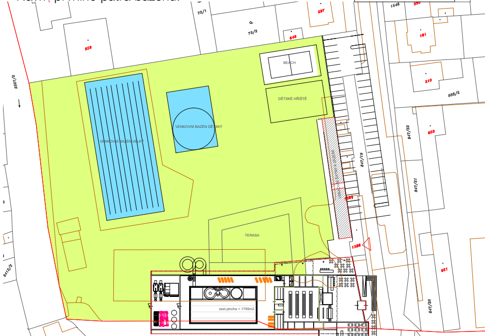
Návrh celkové situace koupaliště a krytého bazénu.
